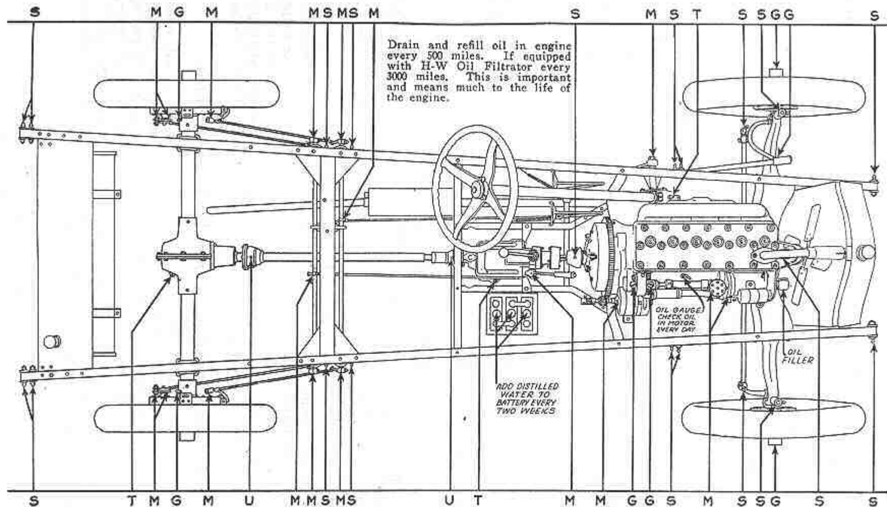
Fig. 85—Lubrication Chart
